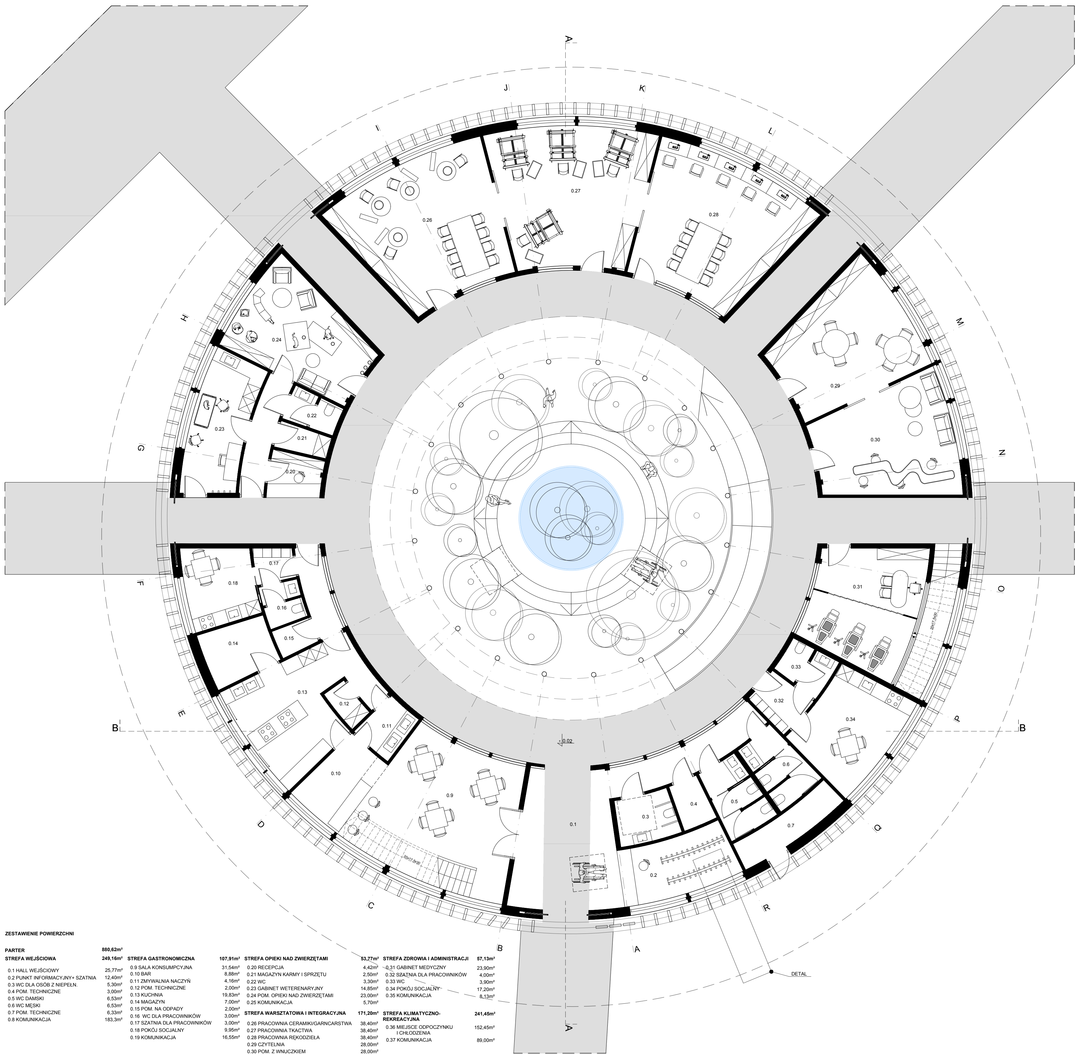
RZUT PARTERU 1:100
