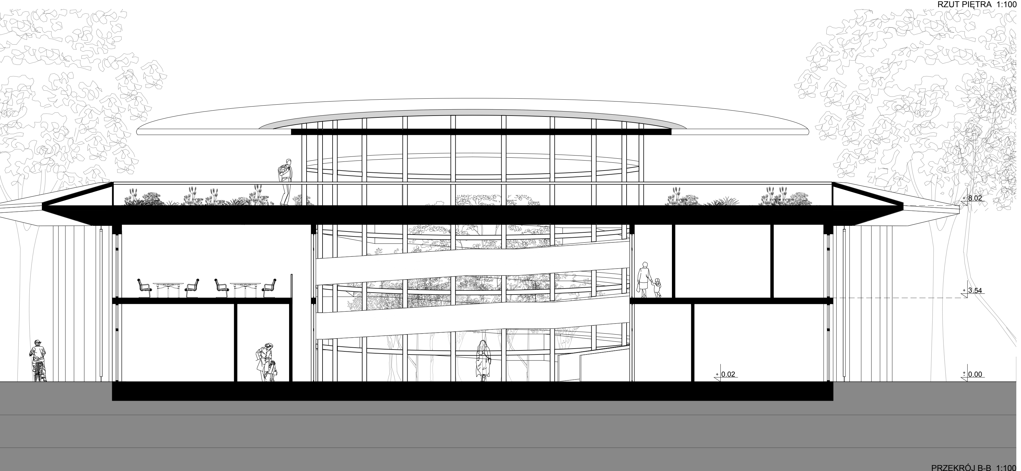
PRZĘKRÓJ B-B 1:100
