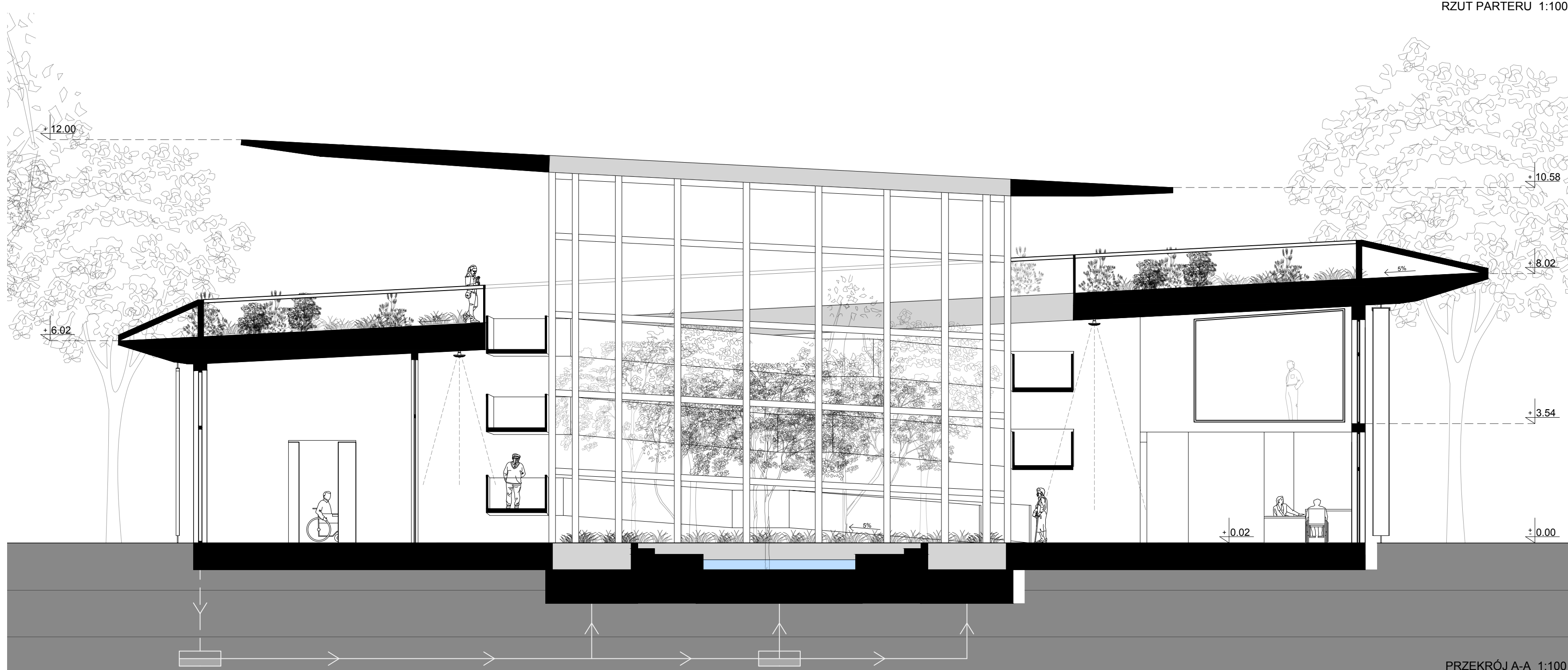
PRZĘKRÓJ A-A 1:100
