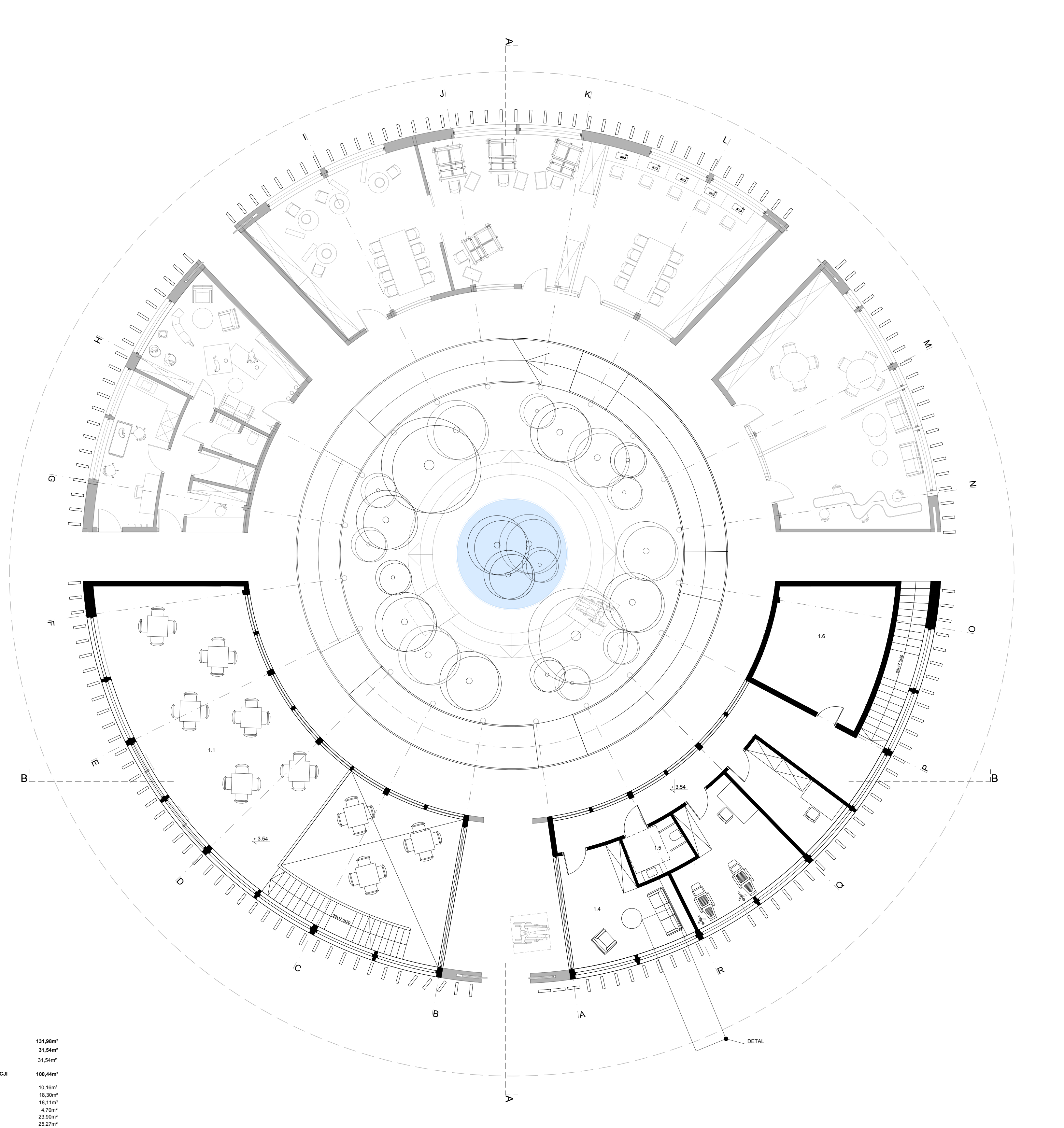
RZUT PIĘTRA 1:100
