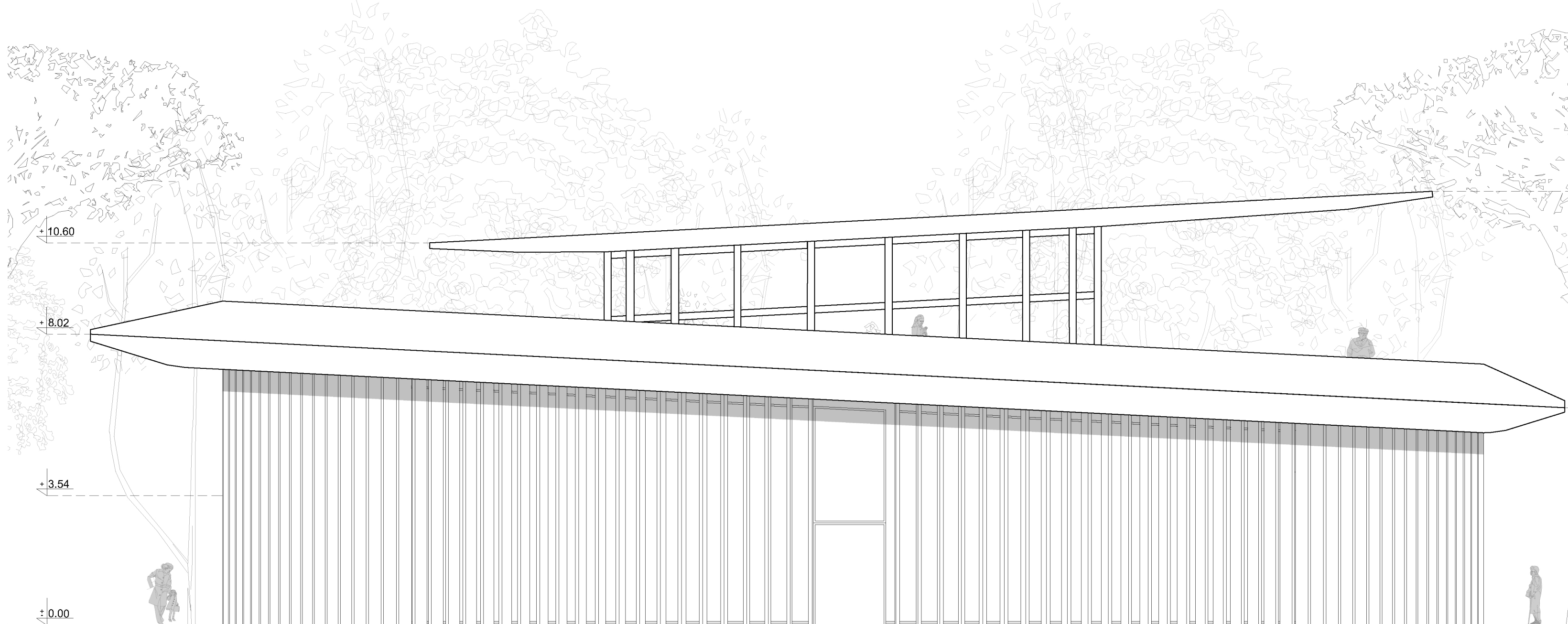
ELEWACJA WSCHODNIA 1:100
