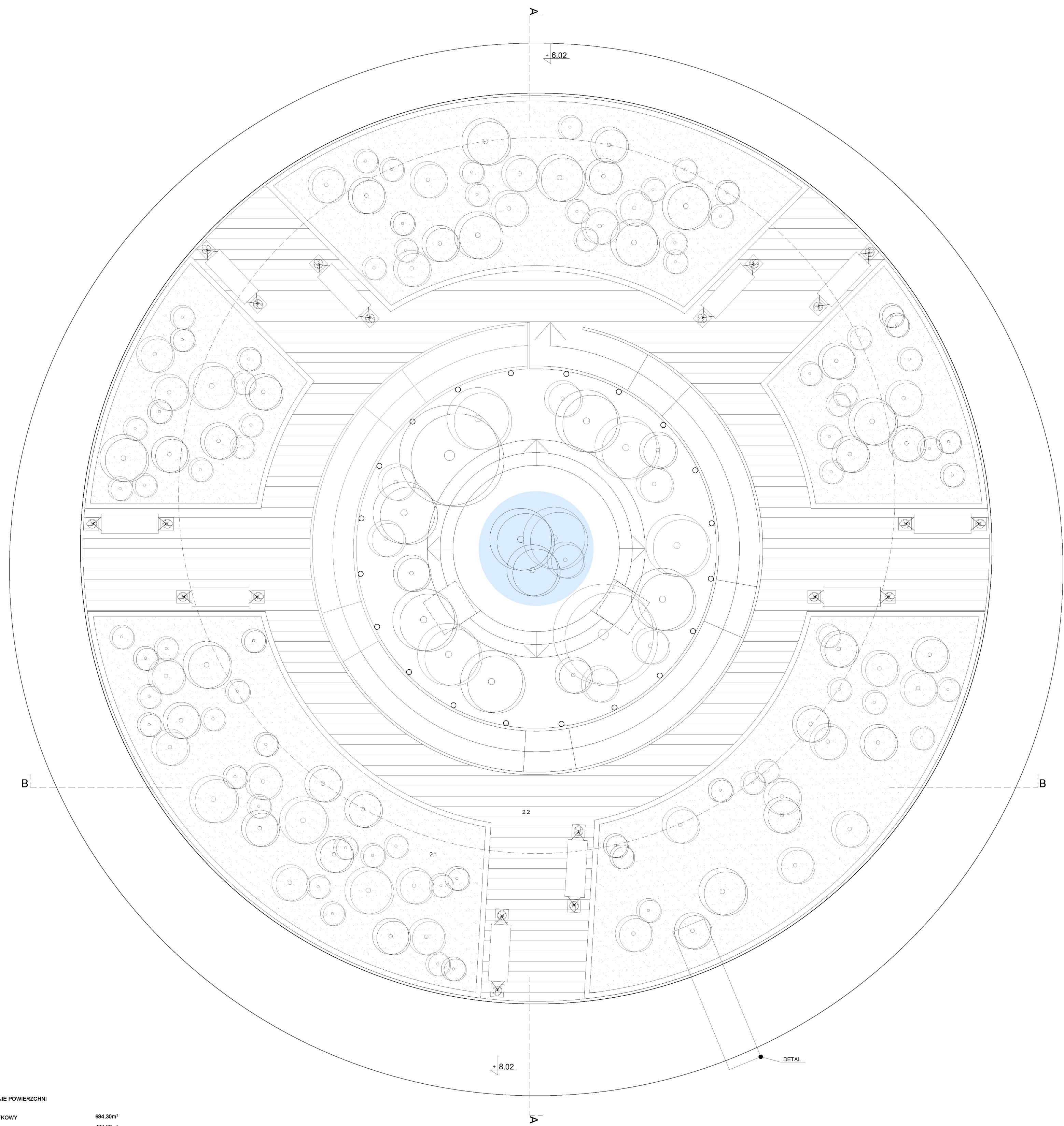
RZUT DACHU 1:100
