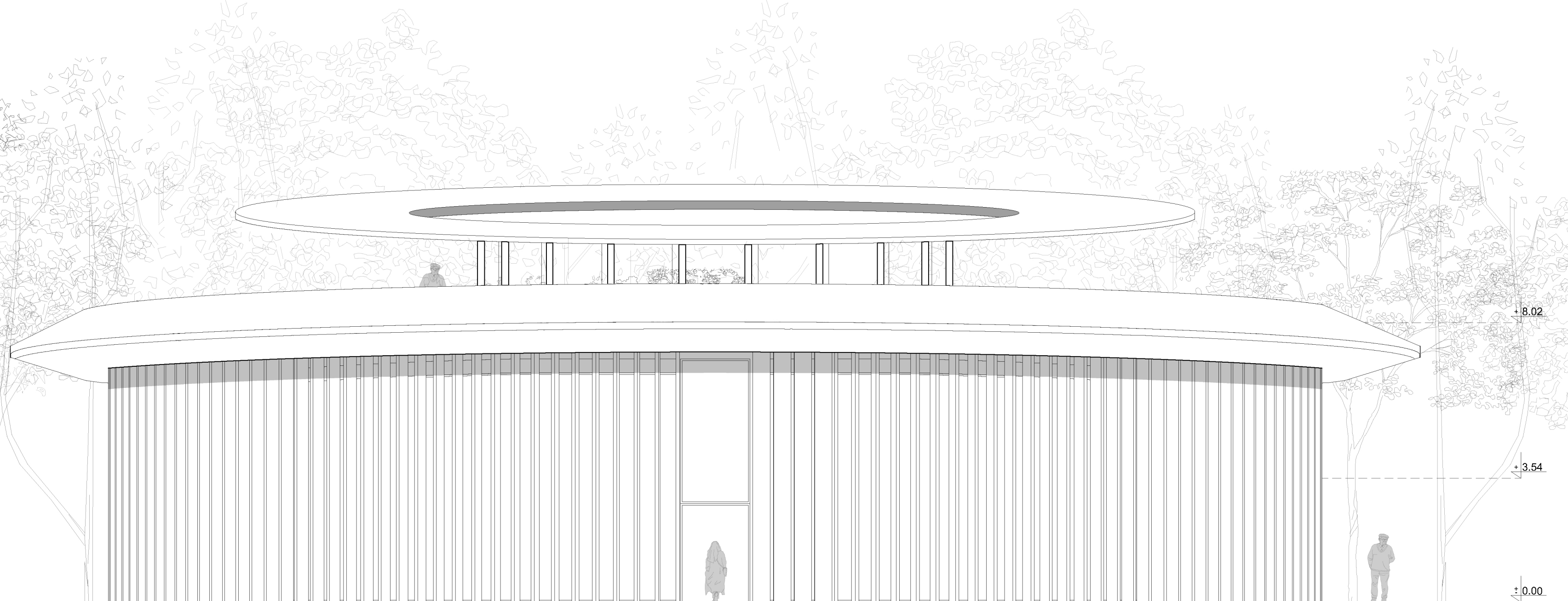
ELEWACJA POŁUDNIOWA 1:100
